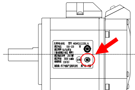
ブラシレスモータ MINAS-BL KV シリーズ (フランジサイズ 60 mm 角、80 mm 角)
